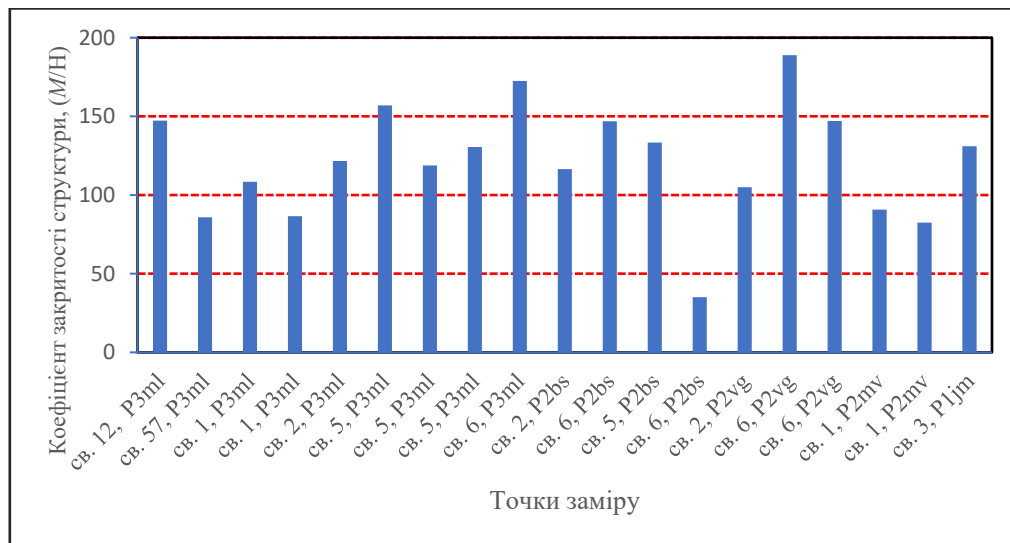
Рис. 5. Ступінь закритості структур Пнівського нафтового родовища
