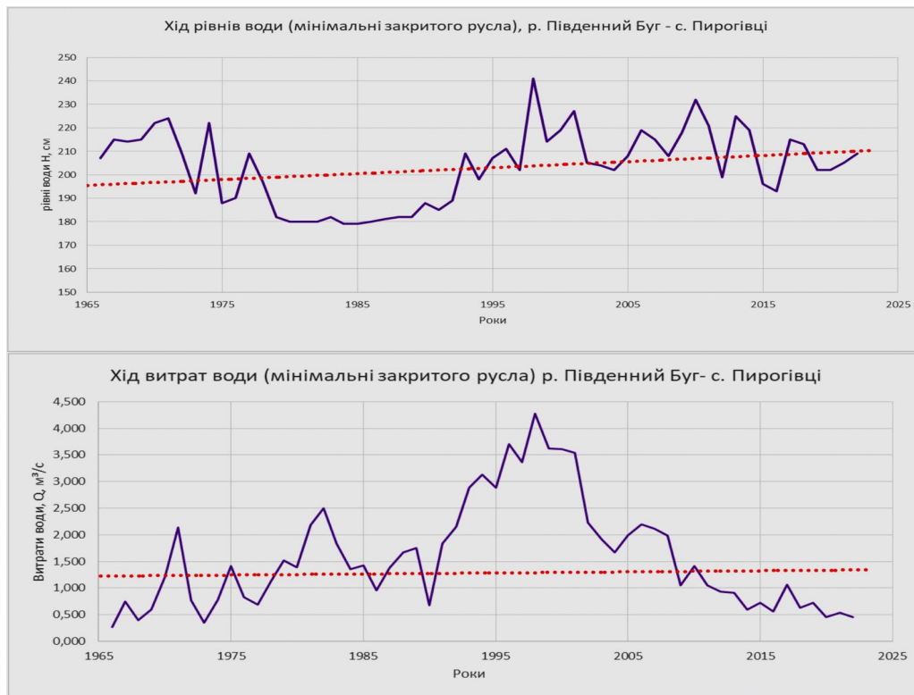
Рис. 6. Суміщення графіків ходу мінімальних рівнів та витрат (закритого періоду русла) р. Південний Буг – с. Пирогівці за весь період спостережень
