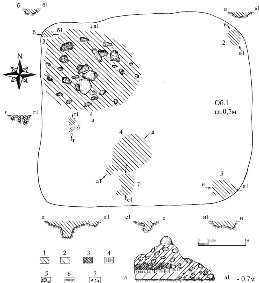
Рис. 3. Винники-Лазки (2016 р.). План долівки житла (об'єкт 1): 1 – гумусоване заповнення об'єктів; 2 – слабогумусоване заповнення об'єктів; 3 – вугілля; 4 – перепалений шар ґрунту; 5 – каміння; 6 – материк; 7 – обмазка.
