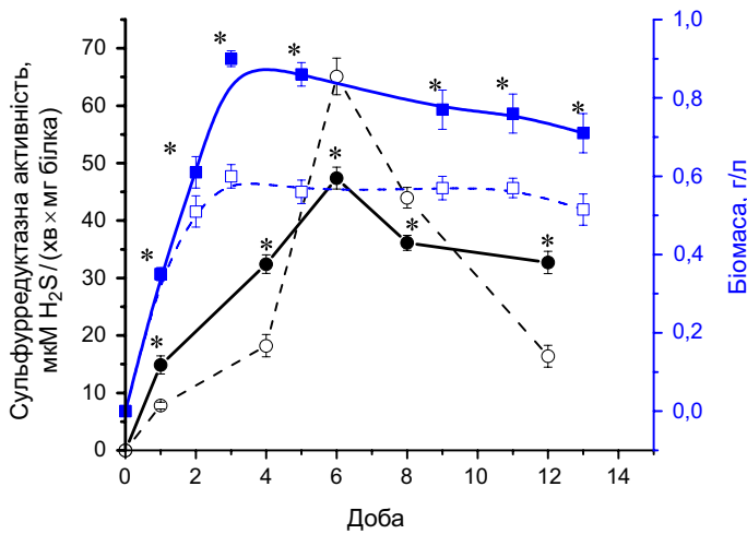
Рис. 3. Нагромадження біомаси та сульфурредуктазна активність бактерій Desulfuromonas sp. YSD S-3 і D. acetoxidans IMB B-7384 у культуральній рідині ( M \pm m , n = 3 )
