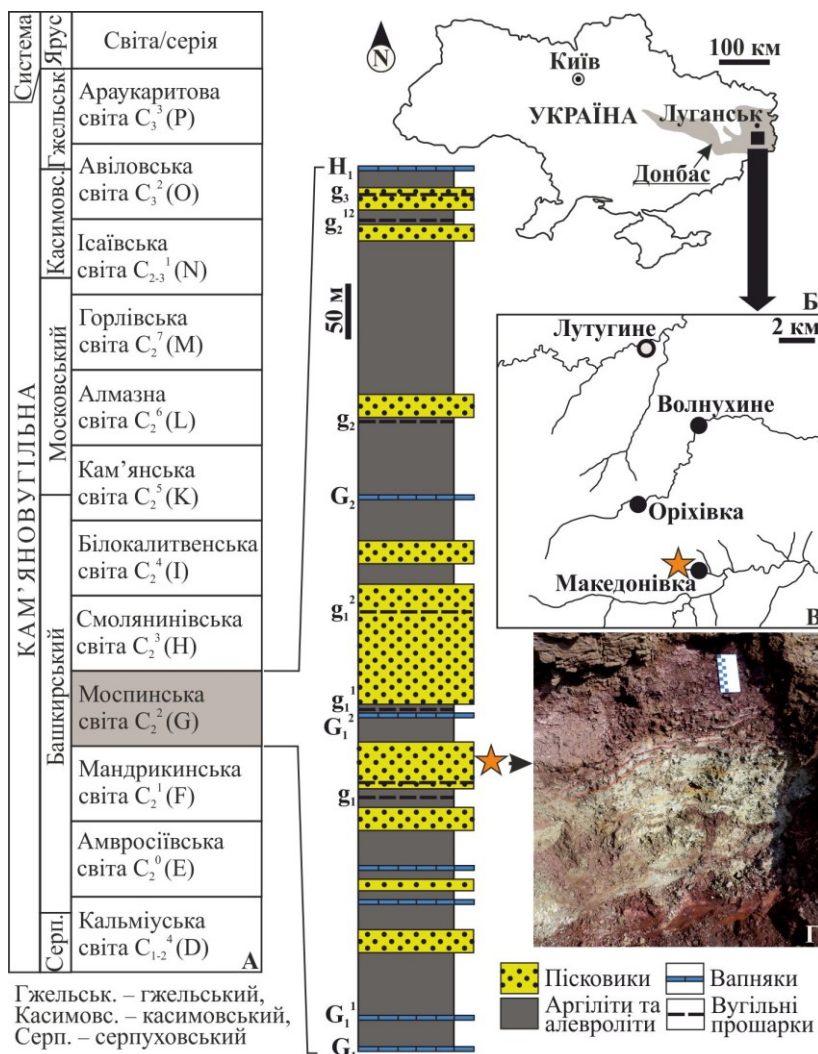
Рис. 1. Розташування та літологічні особливості місцезнаходження решток неморських двостулкових моллюсків: А – стратиграфічне положення моспинської світи та місцезнаходження решток бівальвій; Б, В – географічне розташування місцезнаходження решток двостулкових моллюсків; Г – алевроліти з рештками неморських бівальвій.
