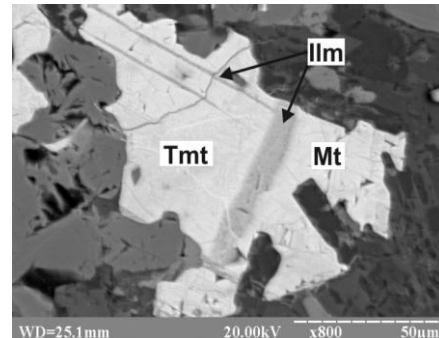
Рис. 6. Зональний індивід залістистої шпінелі зі структурами розпаду твердих розчинів; св. 8 281, гл. 251,5 м (базальт лучичівських верств).
