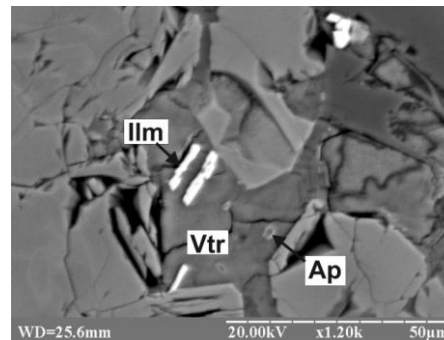
Рис. 8. Ільменіт у вулканічному склі з футляроподібними індивідами апатиту;
