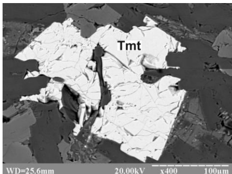
Рис. 7. Зерно однорідного титаномagnetиту без структур розпаду твердих розчинів;
