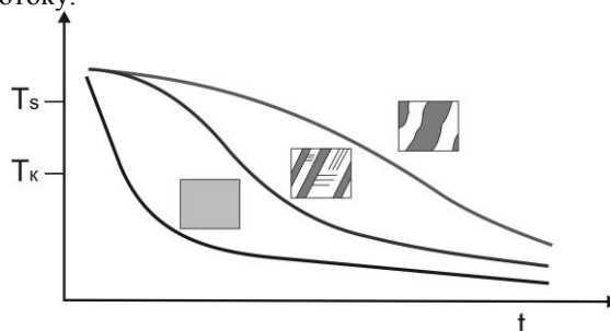
Рис. 13. Схема залежності формування структур розпаду твердих розчинів залістистої шпінелі від часу і температури кристалізації лави ( T_s – температура солідусу; T_k – критична температура; t – час).
