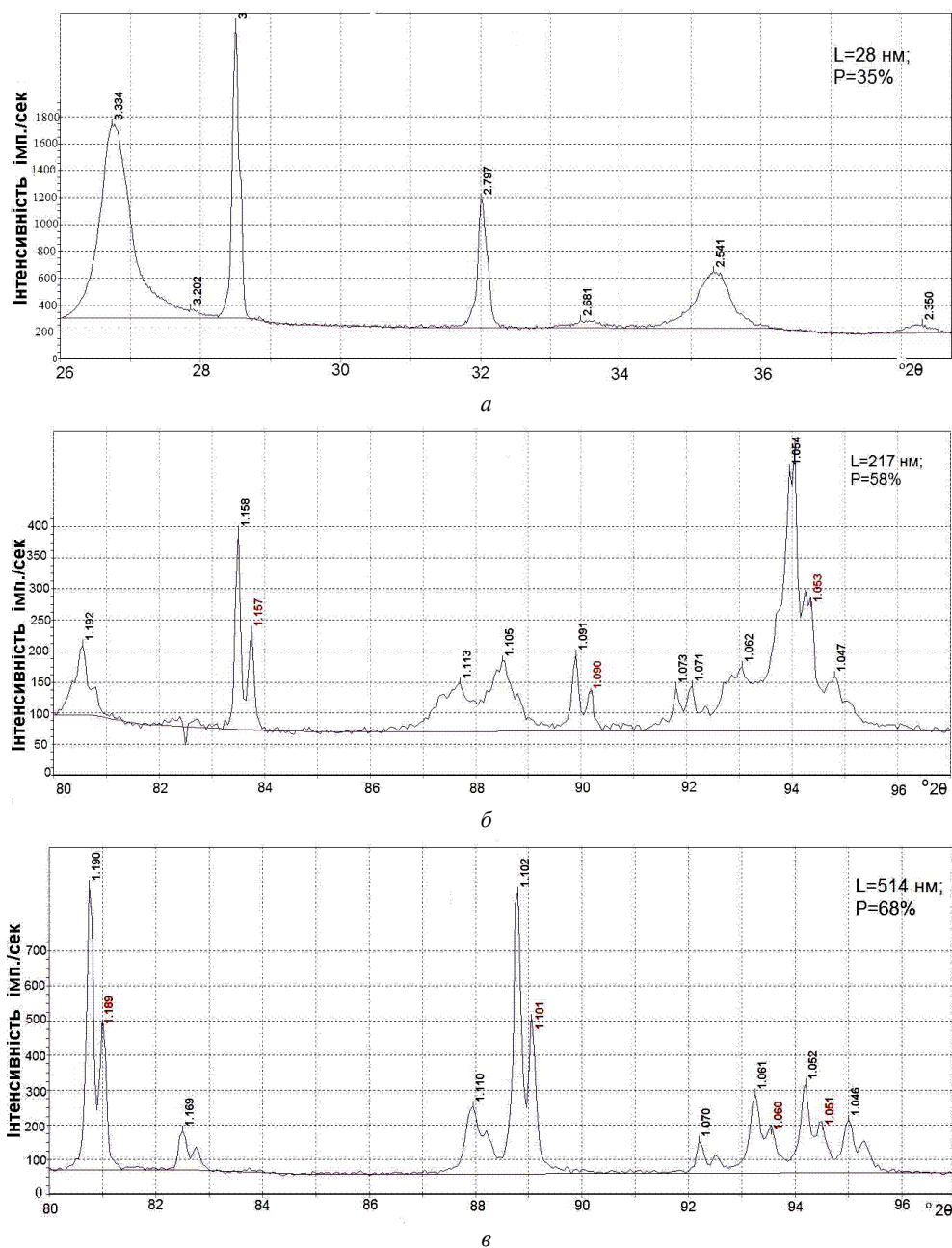
Рис. 3. Дифрактограми циркону з різним ступенем кристалічності, Азовське родовище: а – метаміктний циркон вишневого кольору з лейкократових (св. 19, гл. 79 м) сієнітів; б, в – кристалічний циркон – рожевий (св. 6, гл. 132–134 м) і безбарвний (св. 67, гл. 180,5 м) – з меланократових сієнітів.
