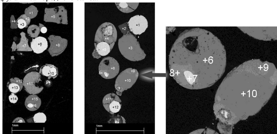
Рис. 7. Внутрішня будова сферул з Якутської алмазонасної провінції, р. Нижня Куанакпа, нижня юра. BSE-зображення.
