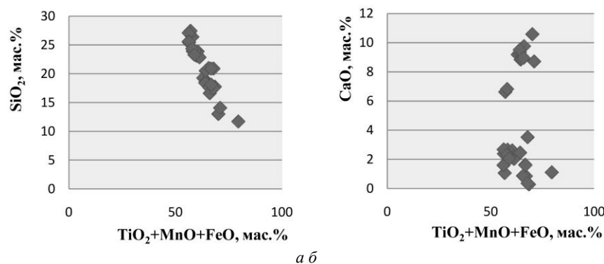
Рис. 14. Залежність між вмістом суми TiO_2+MnO+FeO та кремнеземом (а) і кальцієм (б) у склі ТМЗС-СФ.
