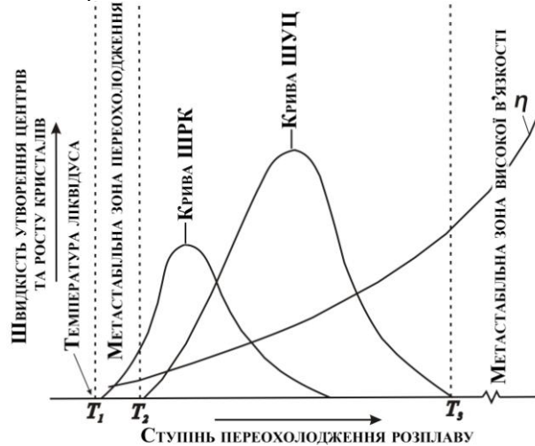
Рис. 6. Діаграма характеру кристалізації силікатного розплаву для випадку задовільної та мінімальної кристалічної здатності, за [3].
