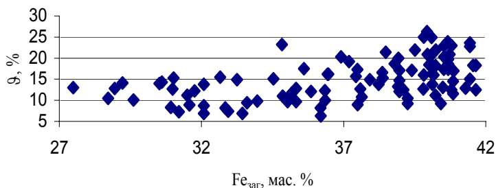
Рис. 10. Характер залежності між показниками втрат заліза у відходах збагачення \theta і загальним вмістом заліза в складі руди Fe_{\text{заг}} .
