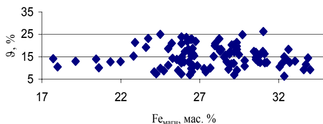
Рис. 9. Характер залежності між показниками втрат заліза у відходах збагачення \theta і вмісту в руді заліза, яке є в складі магнетиту, Fe_{\text{магн}} .
