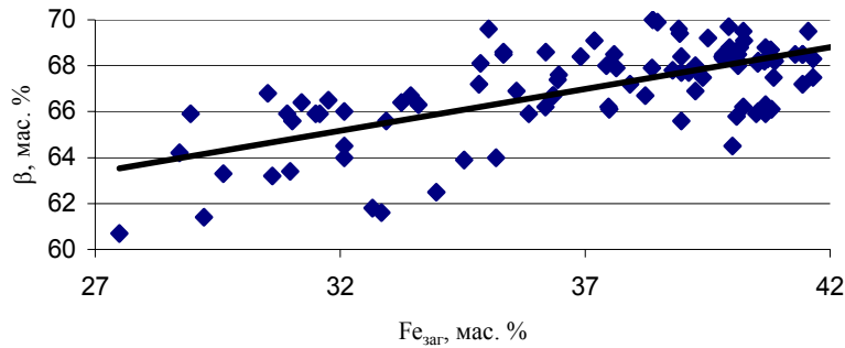
Рис. 3. Характер залежності між показниками загального вмісту заліза в концентраті \beta і загального вмісту заліза в руді Fe_{заг} .
