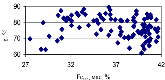
Рис. 8. Характер залежності між показниками вилучення заліза до концентрату \epsilon і загальним вмістом заліза в складі руди Fe_{\text{заг}} .
