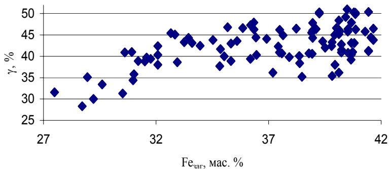
Рис. 6. Характер залежності між показниками виходу концентрату \gamma і загальним вмістом заліза у складі руди Fe_{\text{заг}} .
