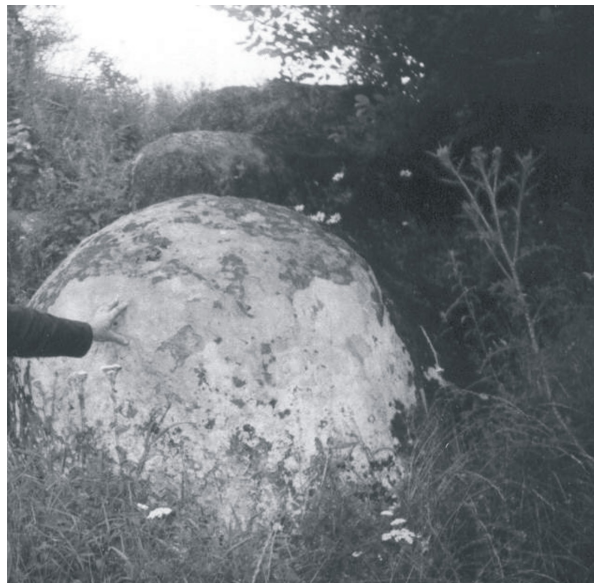
Рис. 2. Піщана конкреція ямненської світи.
