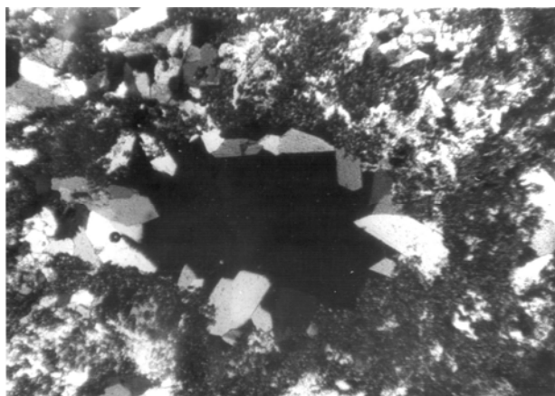
Рис. 4. Гніздоподібне виділення крупнозернистого алуніту серед мікрокварц-алунітової основної маси. Кар'єр Моломко, шліф, ніколі +, \times 70 .
