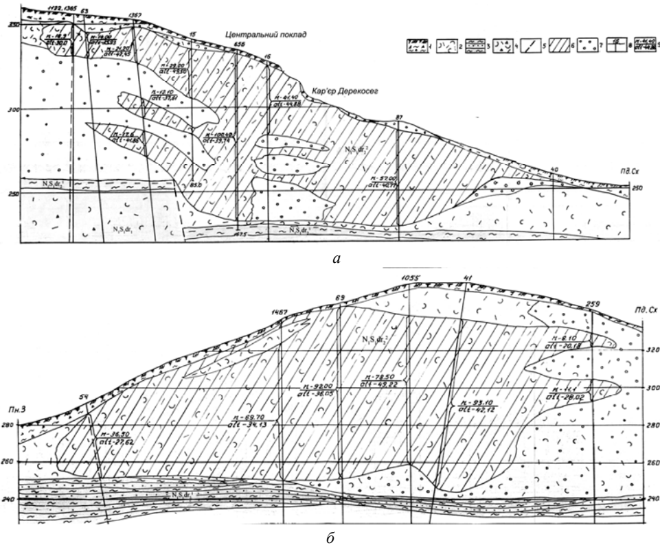
Рис. 1. Геологічні розрізи Берєгівського родовища алунітових руд ділянок кар'єрів Дерекосег (а) та Моломко (центральный поклад) (б):
