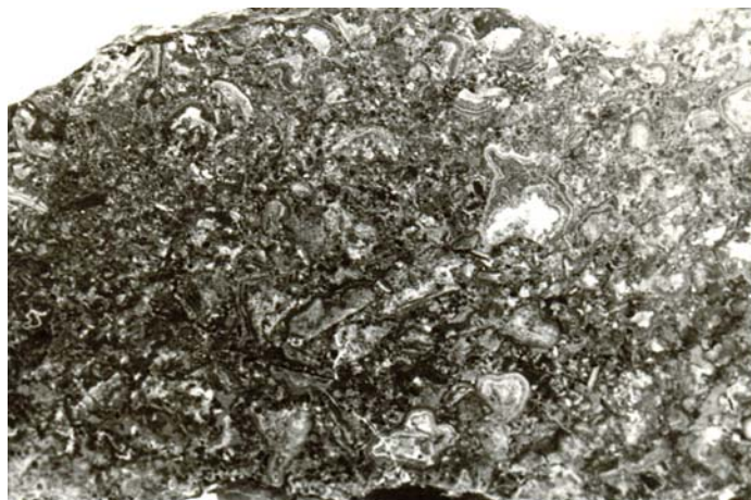
Рис. 1. Брекчієва текстура руди. Помітні уламки концентрично-зонального сфалериту. Полірований штуф.
