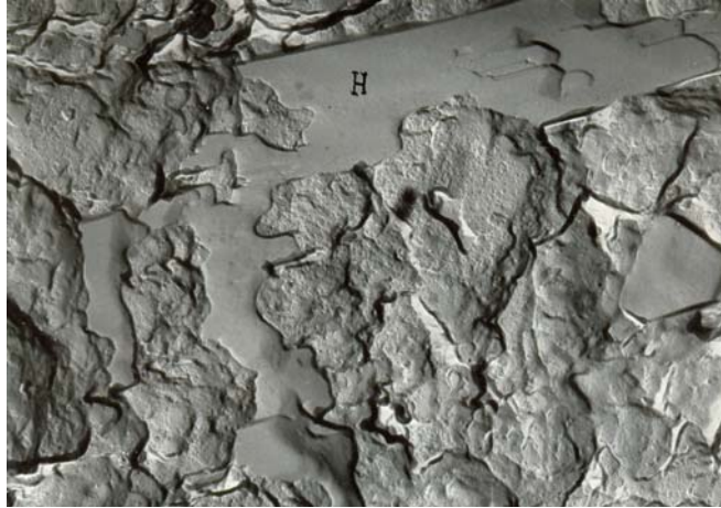
Рис. 5. Корозійне зростання гіпсу (Н) зі сфалеритом. Вугільна репліка, \times 28\ 000 .
