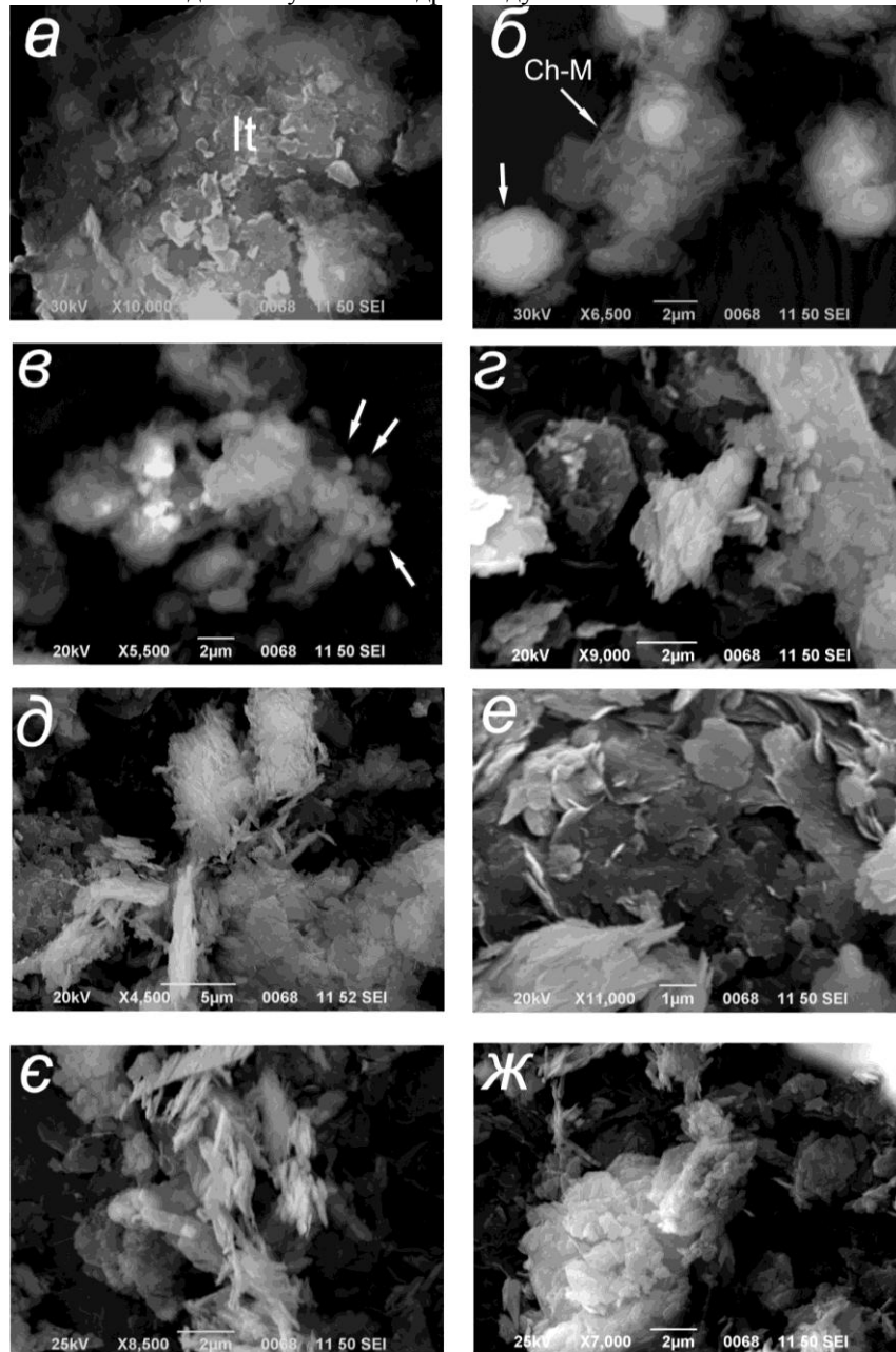
Рис. 5. Електронно-мікроскопічні знімки н. з. кам'яної солі
