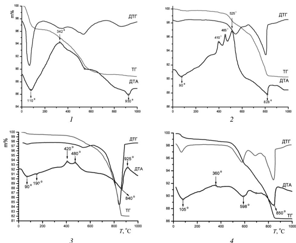
Рис. 4. Криві нагрівання та втрати маси н. з. порід соленосних формацій ДДЗ (фракція до 0,004 мм).
