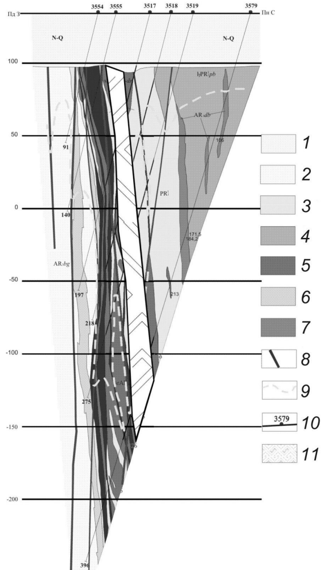
Рис. 2. Положення зони сульфідизації в південній частині Капітанівського ультрабазитового масиву. Розріз по лінії 3554–3579, масштаб 1:3 000 (основа розрізу – за матеріалами ПГЕ ПДРГП Північгеологія).
