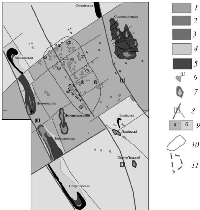
Рис. 1. Схема розташування метамафіт-ультрамафітових структур у центральній частині Голованівського гравімаксимуму (за матеріалами ІПГЕ ПДРГП Північгеологія з доповненнями).
