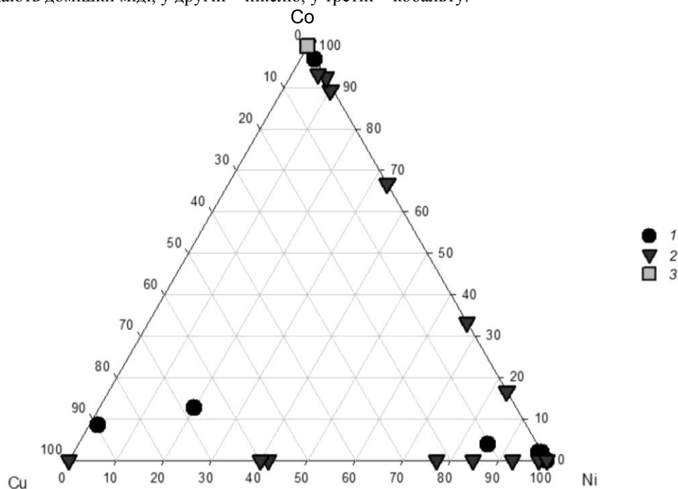
Рис. 4. Розподіл вмісту домішок Ni, Co і Cu в піриті мідно-нікелевих руд норильських родовищ (1), Капітанівського родовища (2) та родовищ Садбері (3).
