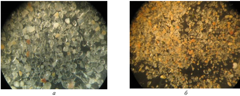
Рис. 11. Фракції розміром 0,25–0,50 ( a ) і 0,10–0,25 мм ( б ) (верхній карниз). Зерна кварцу прозорі, білі, уламки цегли – жовті, червонуваті. Сфотографовано в 5 % HCl.
