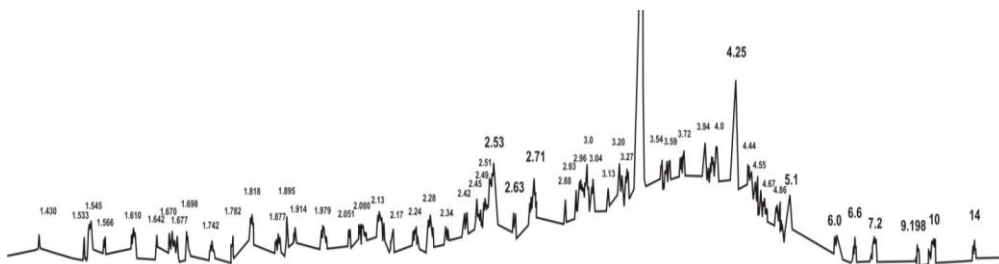
Рис. 12. Рентгенодифрактограма пелітової фракції (< 0,01 мм) породи з верхнього карниза (після обробки HCl).
