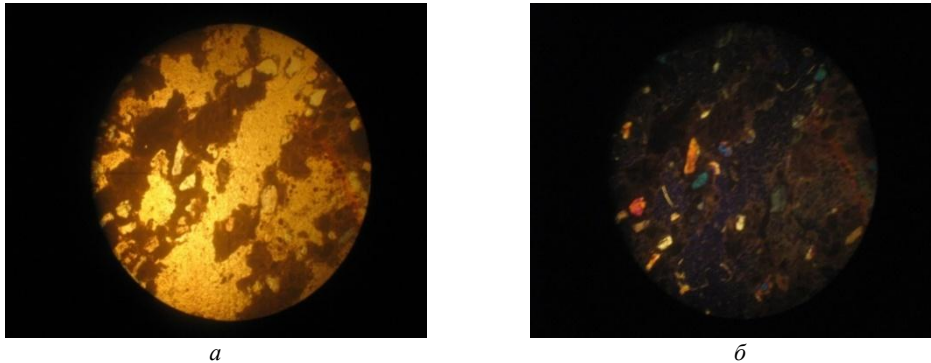
Рис. 10. Штучний камінь з верхнього карниза. Смугаста текстура утворена чергуванням карбонатних (світле) і карбонатно-глинистих виділень: a – без аналізатора, б – з аналізатором; \times 100 .
