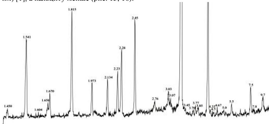
Рис. 15. Рентгенодифрактограма штучного каменю з балаясини балкона універмагу на площі Ринок.
