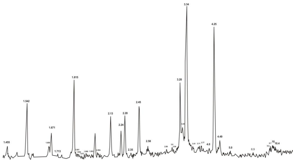
Рис. 13. Рентгенодифрактограма зовнішньої оболонки ("шкірки") породи з верхнього карніза (після обробки HCl).
