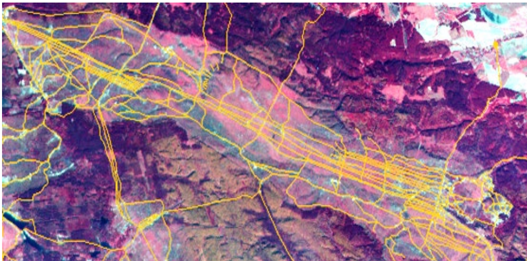
Рис. 5. Колії танкових трас на полях Яворівського полігона (схема дешифрування космоснімка 1985 р.)
