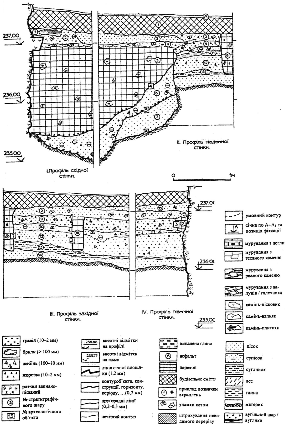
Рис. 2. Стратиграфічні профілі стінок шурфа 1.
