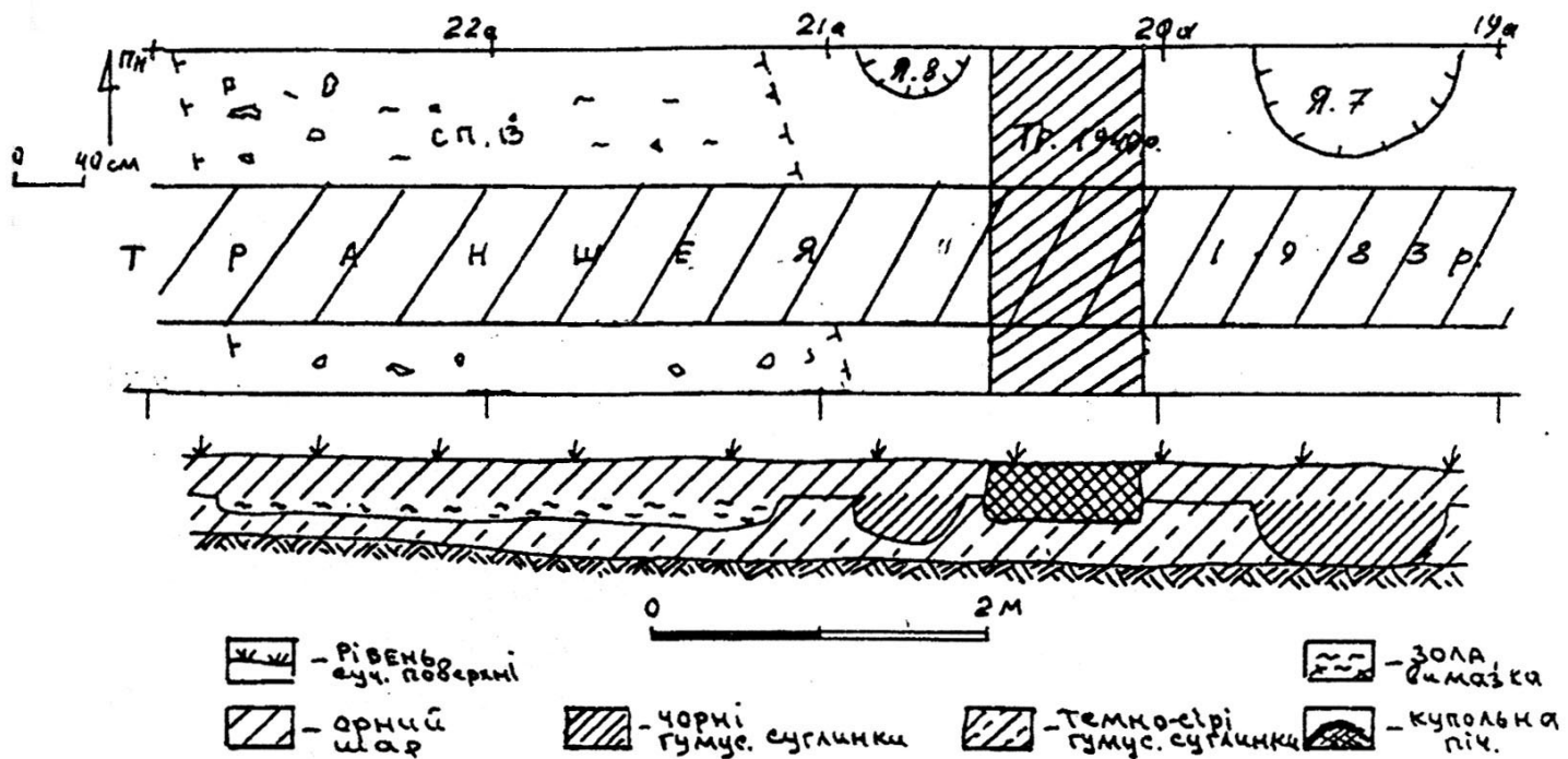
Рис.7. План і профілі споруди № 13 та ям №№ 7 та 8.
