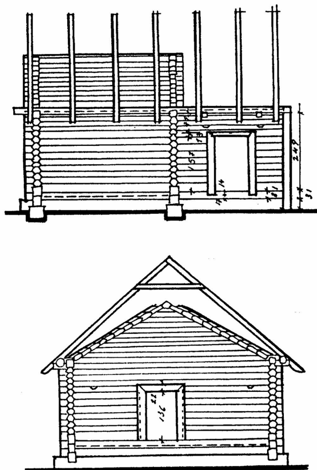
Рис. 2. Зруб комори і сіней середини третьої чверті XIX ст. зі с. Левковичі Овруцького р-ну Житомирської обл. (за Р. Радовичем).
