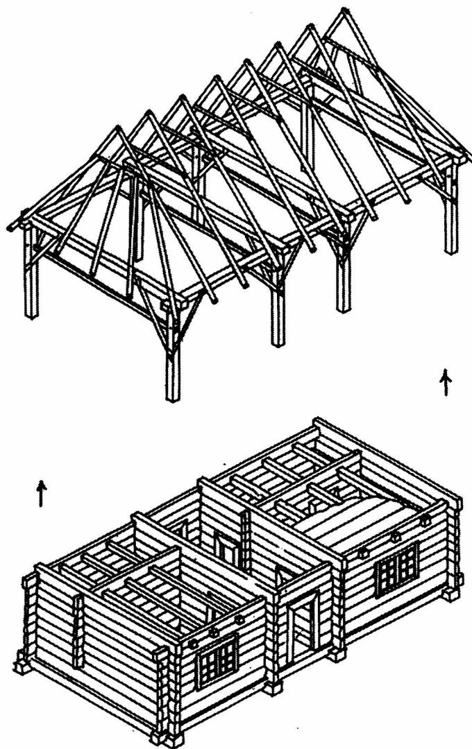
Рис. 4. Хата першої половини – середини ХІХ ст. зі с. Библо Старосамбірського р-ну Львівської обл. (за Р. Рядовичем).
