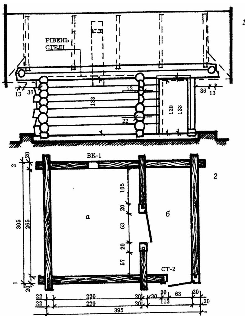
Рис. 3. Стебка середини XIX ст. зі с. Вовчків Поліського р-ну Київської обл. (за Р. Радовичем).
