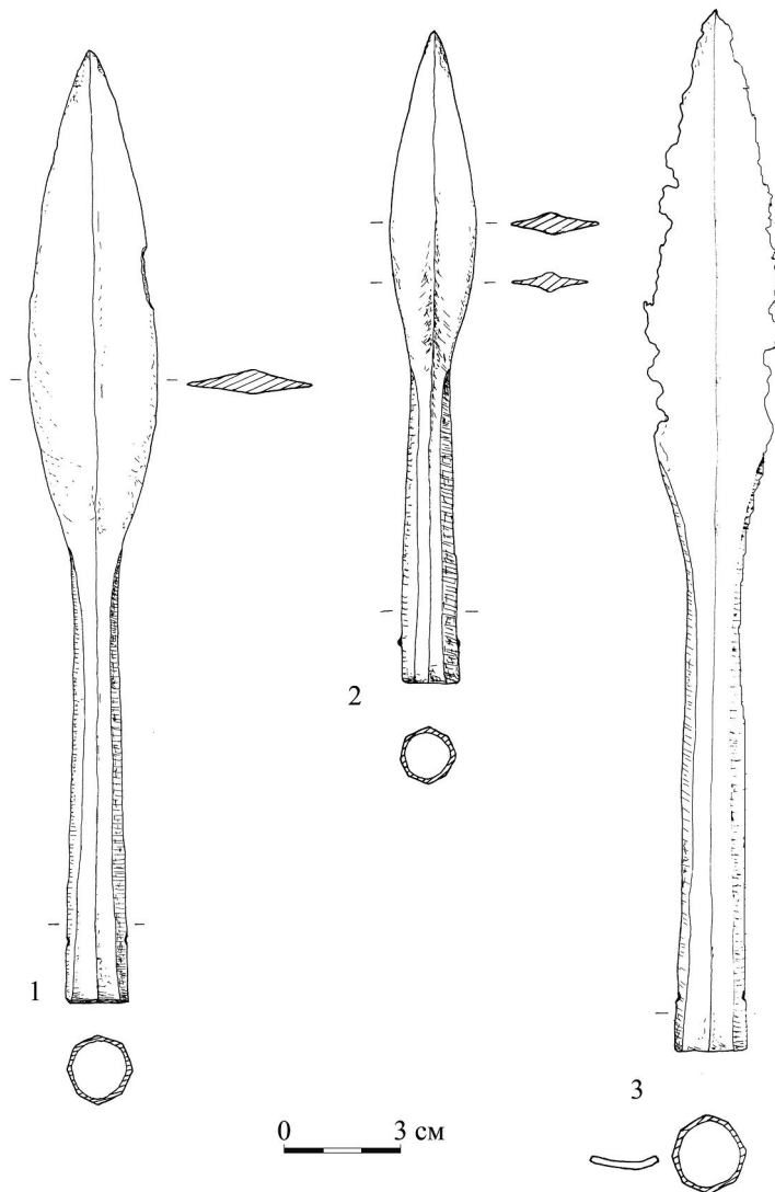
Рис. 3. Наконечники списів із поховання у Вербковіце-Которуві. Fig. 3. Spear pits from burial in Werbkowice-Kotorow.
