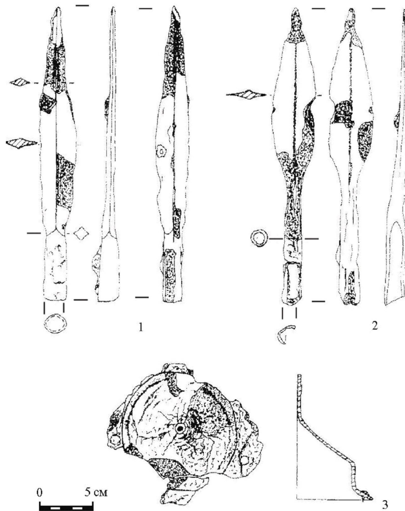
Рис. 2. Бойове спорядження із поховання в Гурі Грабовець. Fig. 2. Weapon and armor from burial in Gura Grabowiec.
