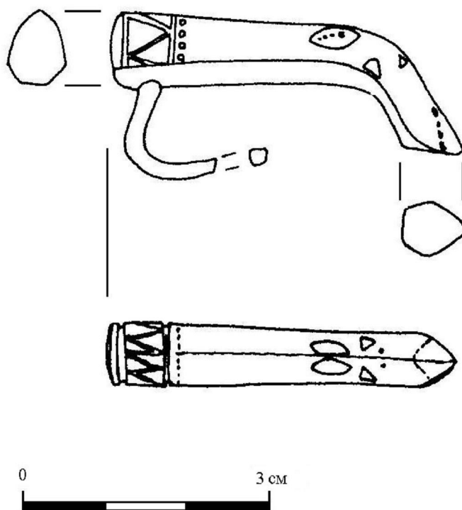
Рис. 4. Дзьобоподібне окуття завершення ремня поясу з Гусинного.
