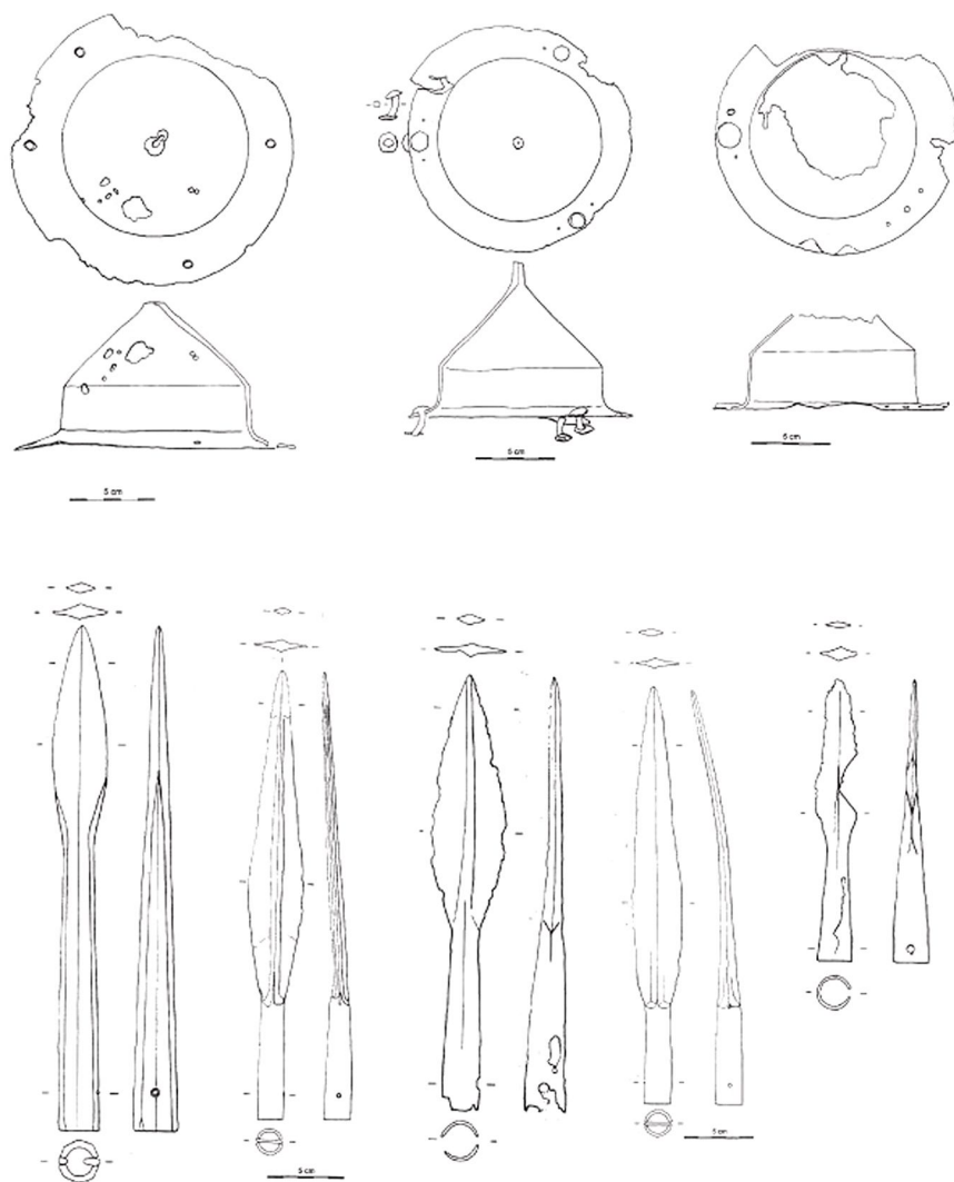
Рис. 1. Бойове спорядження із поховань могильника у Пшеводові. Fig. 1. Weapon and armor from the burials of complex in Przewodow.
