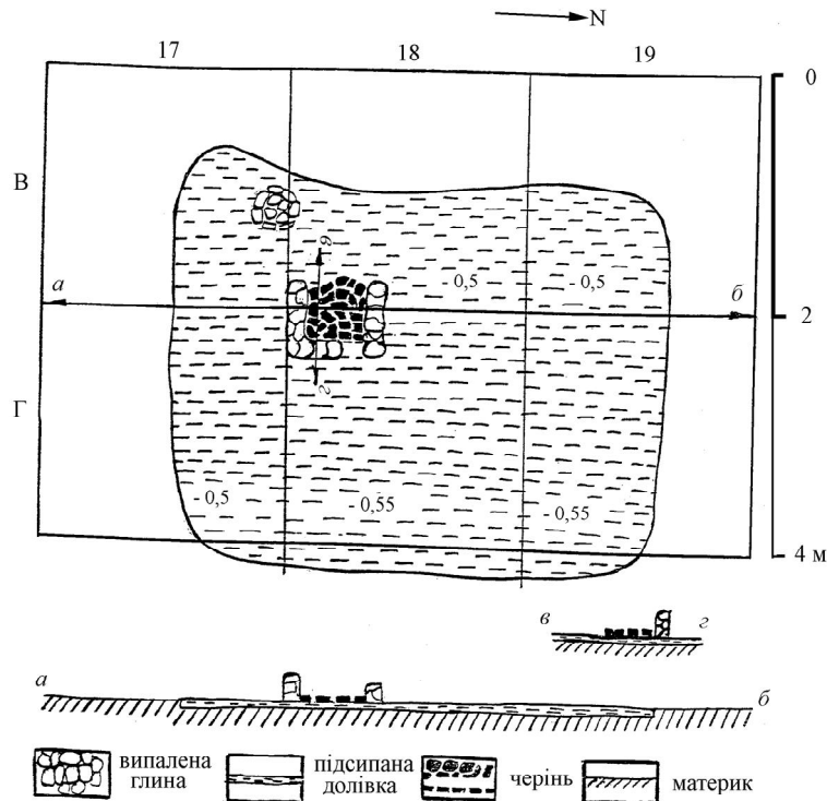
Рис. 2. Стрілки-II, ур. Дубина, 2005. План та переріз наземного житла I. Fig. 2. Strilky-II, Dubyna place, 2005. Plan and section of dwelling I.
