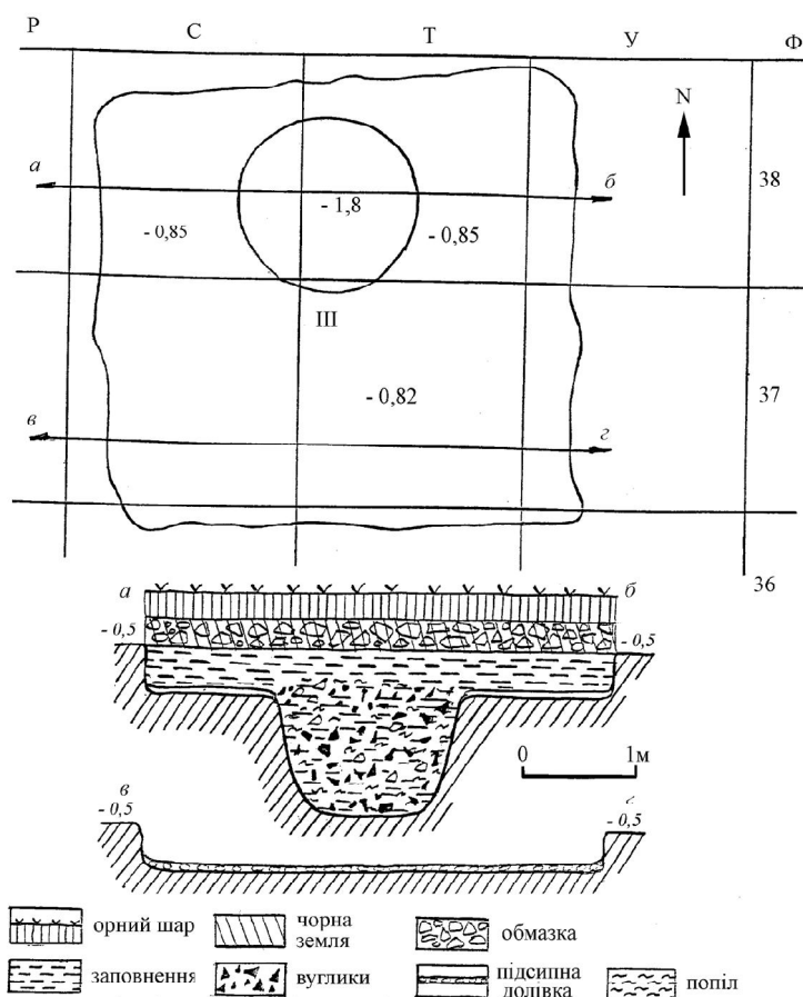
Рис. 4. Стрілки-II, ур. Дубина, 2006. План та переріз житла III. Fig. 4. Strilky-II, Dubyna place, 2006. Plan and section of dwelling III.
