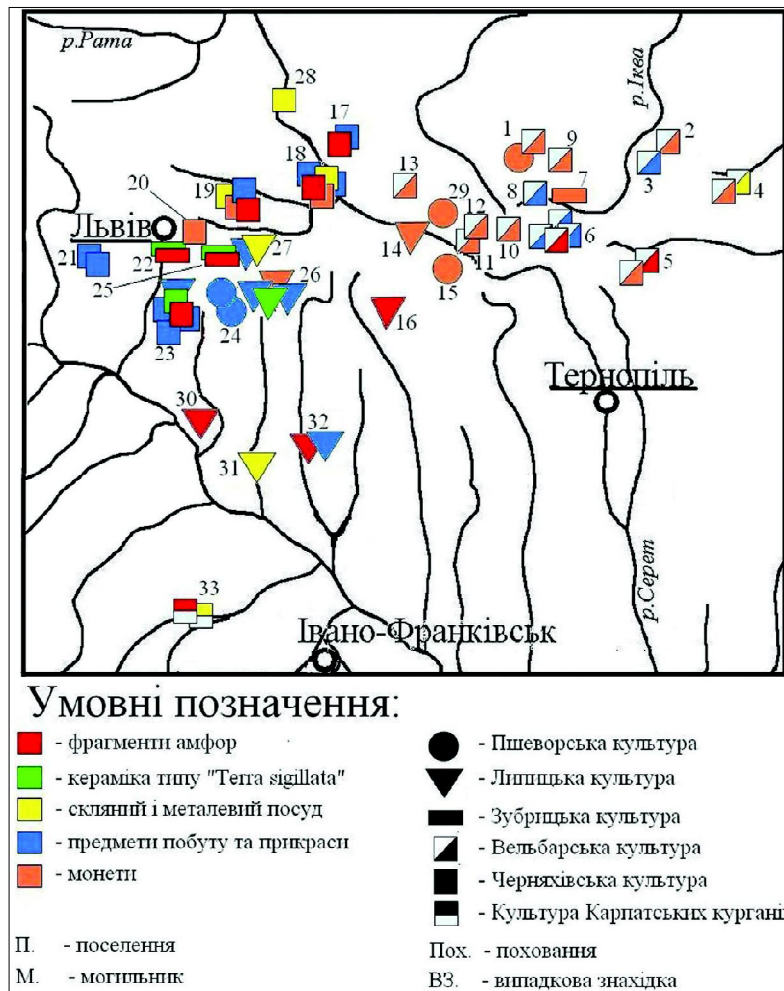
Рис. І. Карта поширення провінційно-римських імпортів на території Північно-Східного Прикарпаття: 1 – Броди (вз.); 2 – Кременець (вз.); 3 – Рудка (пох.); 4 – Вікнини Великі (п.); 5 – Кобылля (п.); 6 – Дудин (п.); 7 – Попівці (п.); 8 – Суховоля (п.); 9 – Бучина (вз.); 10 – Паликорови (вз.); 11 – Орихівчик (вз.); 12 – Малинище (п.); 13 – Йосипівка (п., м.); 14 – Глиняни (вз.); 15 – Почапи (вз.); 16 – Ремезівці (п.); 17 – Ракобовти (п.); 18 – Ріпнів (п.); 19 – Неслухів (п.); 20 – Пікуловичі (вз.); 21 – Наварія (вз.); 22 – Сокільники (п.); 23 – Черепин (п.); 24 – Гринів (м.); 25 – Підберізці (п.); 26 – Звенигород (м., вз.); 27 – Чижиків (пох.); 28 – Кам'янка-Бузька (вз.); 29 – Білий Камінь (вз.); 30 – Заліски (пох.); 31 – Колоколин (пох.); 32 – Верхня Липиця (п., м.); 33 – Нижній Струтинь (м.). Fig. I. Map of imports from Roman provinces on the territory of North-Eastern Carpathians: 1 – Brody; 2 – Kremenets'; 3 – Rudka; 4 – Viknyny Velyki; 5 – Kobyllia; 6 – Dudyn; 7 – Popivci; 8 – Sukhovolia; 9 – Buchyna; 10 – Palykorovy; 11 – Orykhivchuk; 12 – Malynyshche; 13 – Yosypivka; 14 – Hlyniany; 15 – Pochapy; 16 – Remezivtsi; 17 – Rakobovty; 18 – Ripniv; 19 – Neslukhiv; 20 – Pikulovychi; 21 – Navaria; 22 – Sokilnyky; 23 – Cherepyn; 24 – Hryniv; 25 – Pidberizci; 26 – Zvenyhorod; 27 – Chyzykiv; 28 – Kamianka-Buz'ka; 29 – Bilyi Kamin'; 30 – Zalisky; 31 – Kolokolyn; 32 – Verkhnia Lypytsia; 33 – Nyzhnii Strutyn'.
