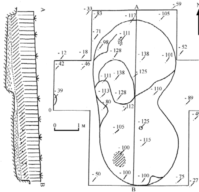
Рис. 3–4. Козина. Профіль і план раньотрипільського об'єкта. Fig. 3–4. Kozyna. Profile and plan of Early Trypilian object.
