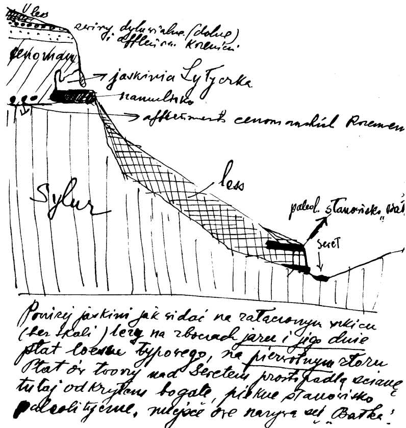
Рис. 6. Геологічний профіль палеолітичної стоянки в с. Лисичники (урочище Балка) на Тернопільщині. Чорновий рисунок Ю. Полянського в листі до С. Круковського від 6 травня 1927 р. (Відділ документації, фонд С. Круковського в Державному археологічному музеї в Варшаві, № 6205).
