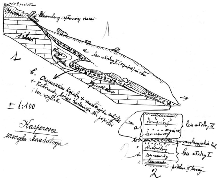
Рис. 9. Геологічний профіль палеолітичної стоянки в урочищі Мандаторія у с. Касперівці при впадінні Серету до Дністра на Тернопільщині. Чорновий рисунок Ю. Полянського в листі до С. Круковського від 10 грудня 1928 р. (Відділ документації, фонд С. Круковського в Державному археологічному музеї в Варшаві, № 6205).
