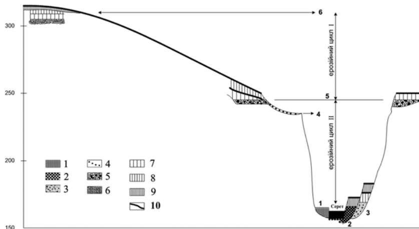
Рис. 4. Схематичний образ терас у нижній течії р. Серет (за Ю. Полянським, 1929): тераси: 1 – перша; 2 – друга; 3 – третя; 4 – четверта; 5 – п’ята; 6 – шоста. Лес: 7 – старший; 8 – молодший I; 9 – молодший II; 10 – викопний/сучасний ґрунт. Виготовила О. Томенюк.
