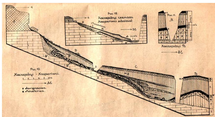
Рис. 10. Геологічний профіль палеолітичної стоянки в с. Касперівці на Тернопільщині. Сторінка з монографії “Подільські етюди” Ю. Полянського. Fig. 10. Geological profile of Paleolithic site in village Kasperivtsi (Ternopil’ region). Page from Y. Polians’kyi’s monography “Podolien Studies”.
