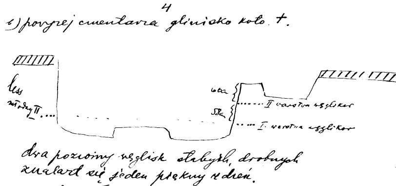
Рис. 8. Геологічний профіль палеолітичної стоянки в Рошневі на Івано-Франківщині. Чорновий рисунок Ю. Полянського в листі до С. Круковського від 6 травня 1927 р. (Відділ документації, фонд С. Круковського в Державному археологічному музеї в Варшаві, № 6205).
