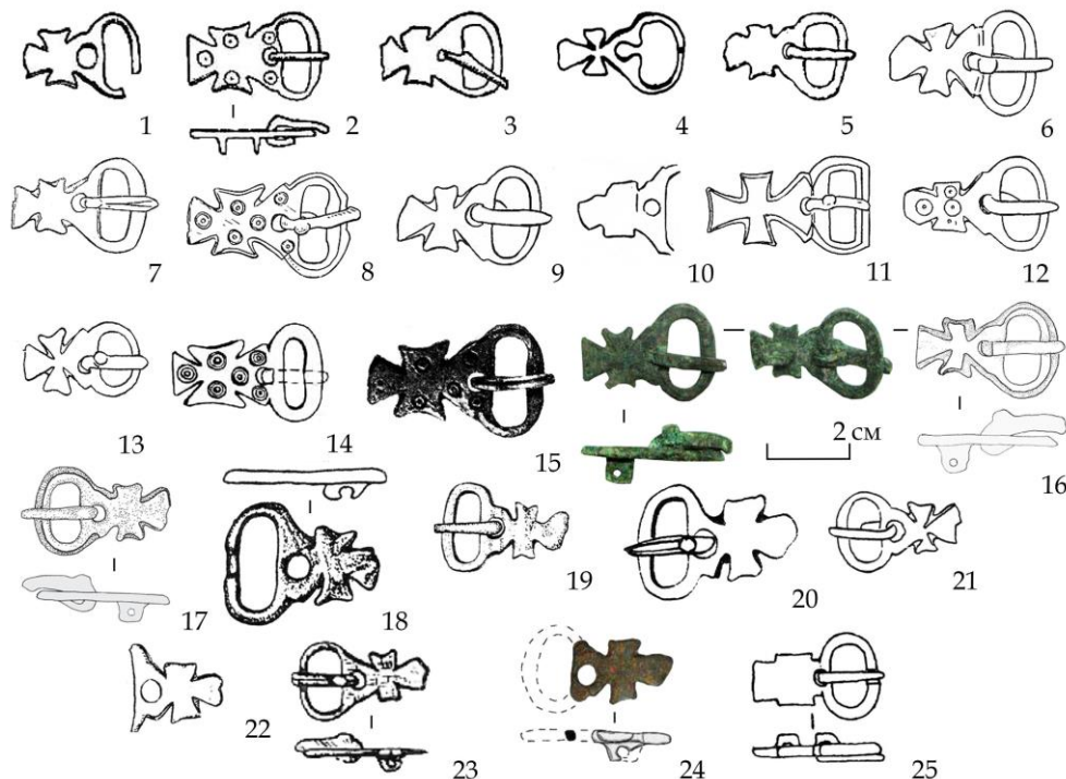
Рис. 7. Візантійські пряжки із щитком хрестоподібної форми із Криму: 1–3 – Херсонес, поховання 20 [Якобсон, 1959, рис. 139, 10–12]; 4 – Аромат, склеп 6 [Лобода, 1976, рис. 5, 29]; 5 – Мале Садове, склеп 6 [Омелькова, 1990, рис. 1, 47]; 6 – Ескі-Кермен, склеп 65 [Айбабин, 1982, рис. 3, 5]; 7 – Ескі-Кермен, склеп 181 [Айбабин, 1982, рис. 4, 8]; 8 – Ескі-Кермен, склеп 257 [Айбабин, 1982, рис. 10, 8]; 9 – Узень-Баш, склеп 3 1958 р. [Айбабин, 1982, рис. 3, 4]; 10 – Узень-Баш, склеп 1 1907 р. [Айбабин, 1982, рис. 3, 8]; 11 – Керч, склеп 52, кістяк 1 [Айбабин, 1982, рис. 3, 15]; 12 – Суук-Су, поховання 53 [Айбабин, 1982, рис. 3, 11]; 13 – Суук-Су, поховання 55 [Айбабин, 1982, рис. 3, 12]; 14 – Суук-Су, склеп 131 [Айбабин, Хайрединова, 2017, рис. 123, 26]; 15 – Чуфут-Кале, склеп 43 [Кропоткин, 1965, рис. 44, 5]; 16, 17 – Алмалик-Дере, склеп 177 2005 р. [Maćczyńska, Gercen, Ivanova, Černyš, Lukin, Urbaniak, Bemmman, Schneider, Jakubczyk, 2016, Taf. 251, 2; 255, 2]; 18 – Скалисте, склеп 371 [Веймарн, Айбабин, 1993, рис. 57, 1]; 19 – Скалисте, склеп 381 [Веймарн, Айбабин, 1993, рис. 60, 18]; 20 – Скалисте, склеп 400 [Веймарн, Айбабин, 1993, рис. 64, 37]; 21 – Скалисте, склеп 625 [Веймарн, Айбабин, 1993, рис. 103, 4]; 22 – Скалисте, окрема знахідка [Веймарн, Айбабин, 1993, рис. 107, 16]; 23 – Лучисте, склеп 95, поховання 3 [Schulze-Dörrlamm, 2009, Abb. 70, 4]; 24 – Мангупський палац [Науменко, Набоков, 2021, рис. 1, 3]; 25 – Сугдея, розкоп V в портовій частині [Майко, 2020, рис. 126, 5]. 14, 20 – без масштабу.
