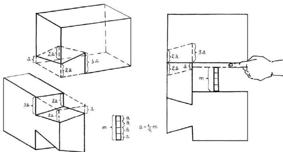
Рис. 2. Влаштування двосторонньої врубки типу “риб’ячий хвіст” без лишку
