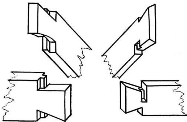
Рис. 7. Кутові врубки типу “риб’ячий хвіст” з прихованим зубом на Підляшші (за С. Стащак)
