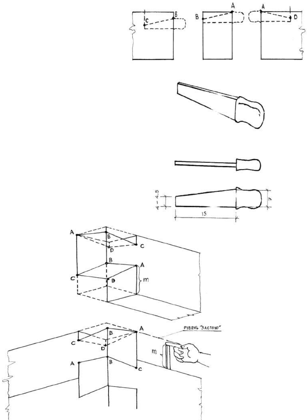
Рис. 3. Влаштування односторонньої врубки типу "риб'ячий хвіст"
