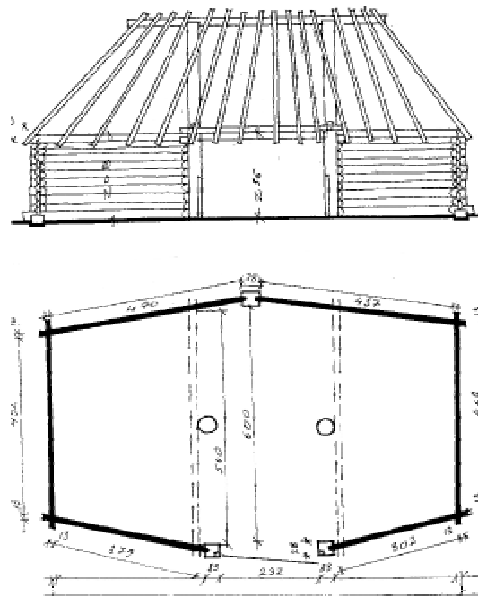
Іл. 2. Семигранний "ток", с. Левковичі Овруцького р-ну Житомирської обл.
