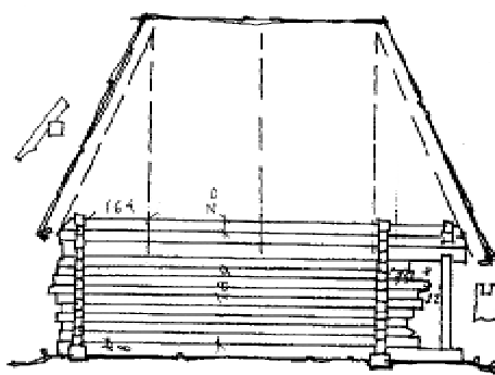
Іл. 5. "Точок" кін. XIX ст., с. Кишин Олевського р-ну Житомирської обл.
