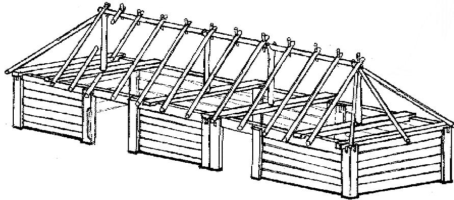
Іл. 6. “Ток” поч. XX ст., с. Червінь Дубровицького р-ну Рівенської обл.
