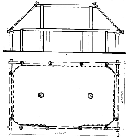
Іл. 4. "Гумно" поч. XX ст., с. Ладижичі колишнього Чорнобильського р-ну Київської обл.
