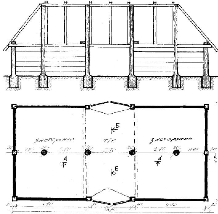
Іл. 1. "Клуня" поч. XX ст., с. Перевали Турійського р-ну Волинської обл.
