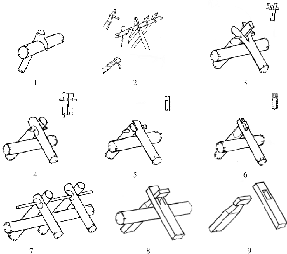
Іл. 7. Конструктивні варіанти “ключин”: 1) “ключина”, виготовлена із стовбура з природною розвилкою; 2) “ключини” із гакоподібним виступаючим кілком (за В. Трацевським); 3–6) “ключини”, попарно з’єднані кілком; 7) “ключини”, нанизані на одну жердину; 8) специфічне кріплення “ключин” (за В. Трацевським); 9) специфічне кріплення “ключин” (за З. Дмоховським)
