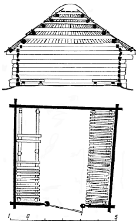
Іл. 17. “Ток”, с. Кишин Олевського р-ну Житомирської обл. (за С. Верговським)
