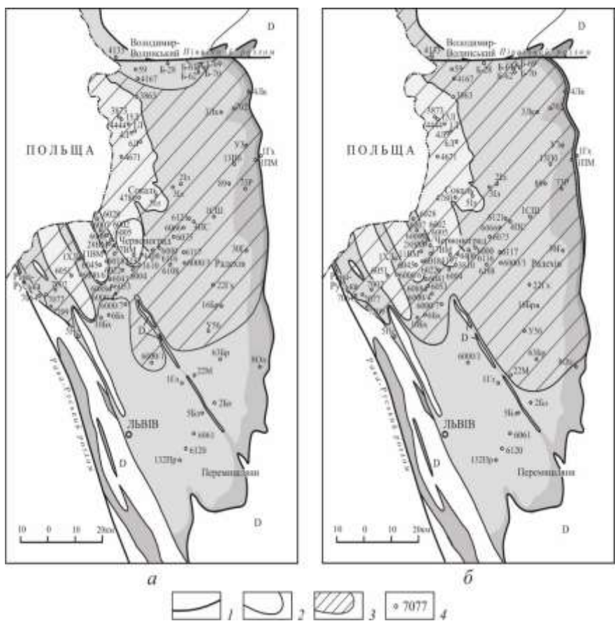
Рис. 3. Схеми поширення світ: а – хорівської, б – куличківської [9]:
