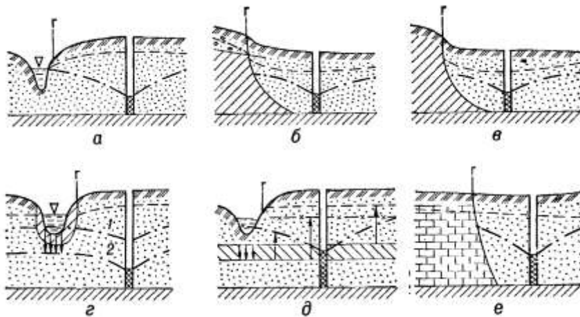
Рис. 1. Умови на межах водоносних горизонтів у плані: z – границя; граничні умови: a – першого роду; b – другого роду ( Q = \text{const} \neq 0 ); c – другого роду ( Q = 0 ); d – третього роду; e – четвертого роду.
