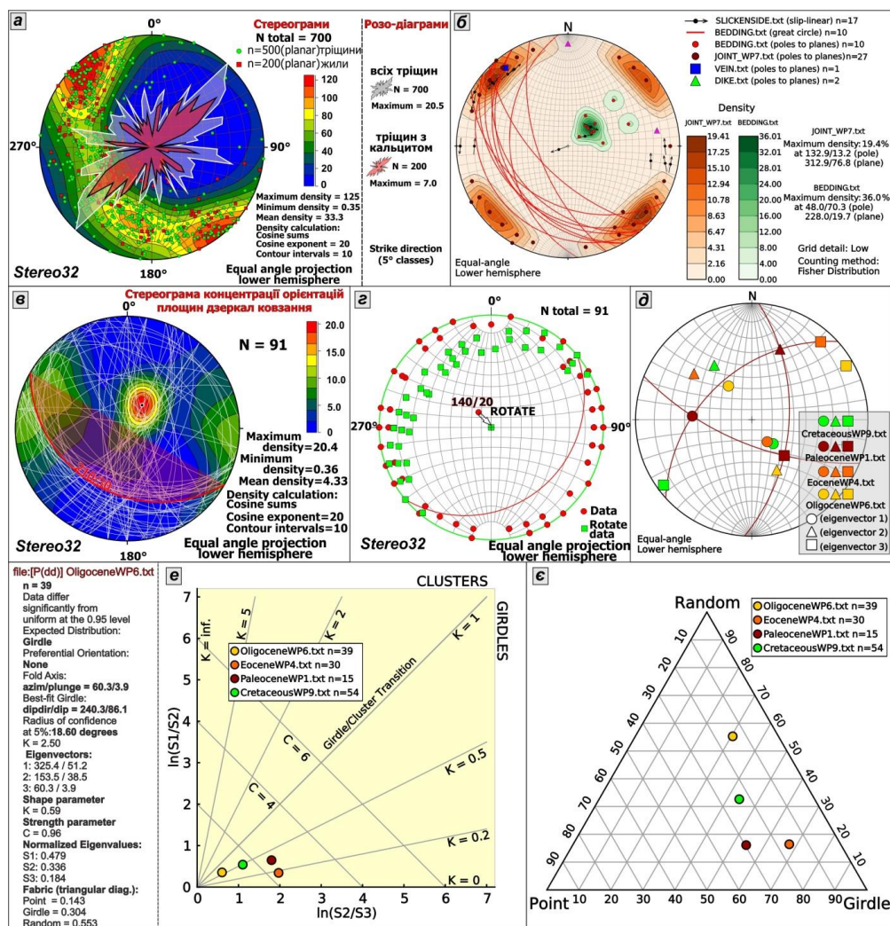
Рис. 3. Комплексні діаграми на прикладі відслонень Скибового покриву, побудовані з допомогою програм Stereonet : a – стереограма полюсів тріщин та розо-діаграми для тріщин пустих та з мінеральним вповненням на відслоненнях долини р. Опір ( Stereo32 ); б – вектори переміщень по дзеркалах ковзання, стереограми полюсів напластування тріщин, карбонатних жил, кластичних дайок у верхній течії р. Сукіль ( OpenStereo ); в – стереограма концентрації орієнтацій площин дзеркал ковзання (р. Сукіль) ( Stereo32 ); з – структурні дані за сучасного
