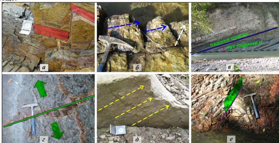
Рис.1. Приклади найпоширеніших площинних ( а-с ) та лінійних ( д, е ) структур у відслоненнях Скибового покриву Українських Карпат ( а – тріщини; б – дзеркала ковзання; в – шаруватість порід; г – кластична дайка у палеогенових відкладах; д – риси на площині дзеркала ковзання; е – шарнір та крила складки)
