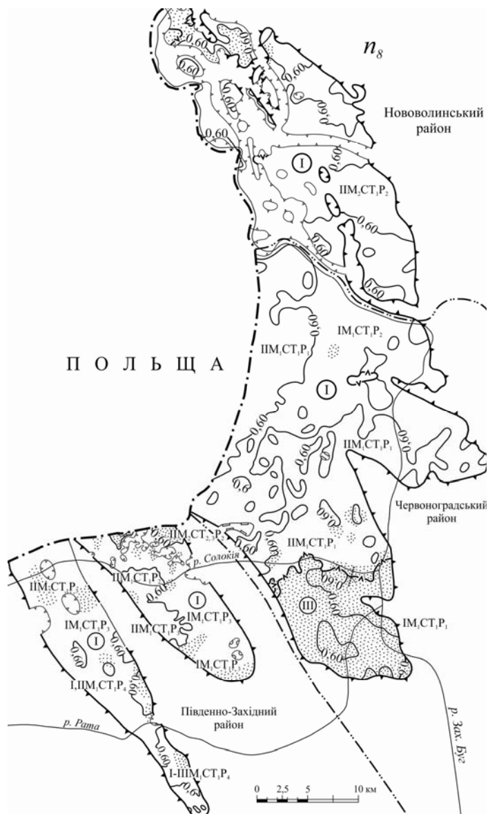
Рис. 4. Карта морфології вугільного пласта n_8 Львівсько-Волинського кам'яновугільного басейну (умовні позначення див. рис. 3)
