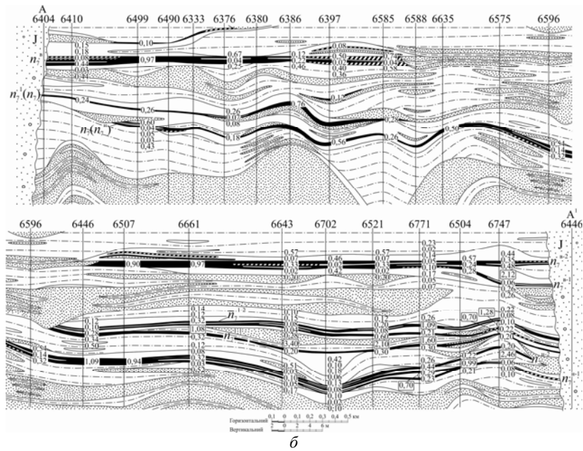
Рис. 3. Карта морфології вугільного пласта n_7^1(n_7) (а) і деталізаційний морфологічний розріз кондиційних пластів вугілля n_7(n_7^H) - n_7^B (б) Тягівського родовища Південно-Західного вугленосного району ЛВБ:
