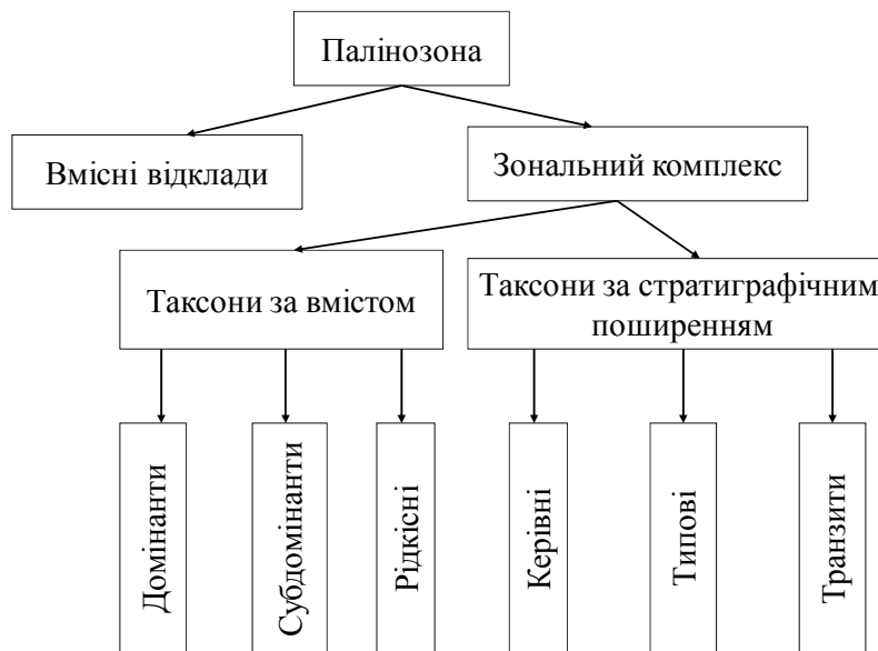
Рис. 2. Структура палінозони
