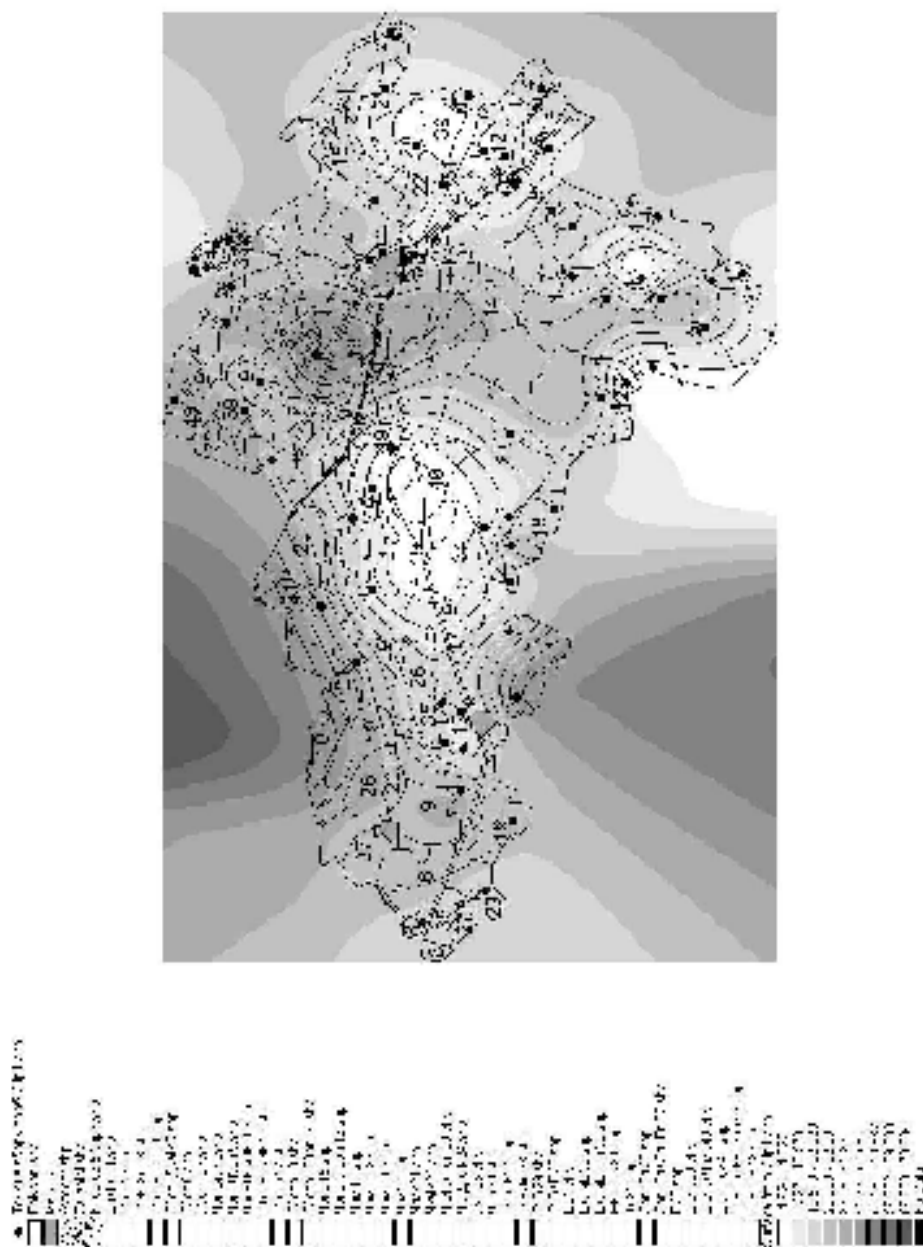
Рис. 6. Картохема забруднення ґрунтів Золочівського р-ну валовим нікелем, мг/кг.
