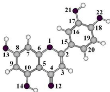
Рис. 5. Оптимальна геометрична будова молекули лутеоліну
