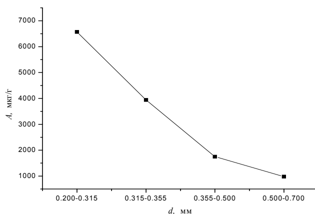
Рис. 1. Залежність сорбційної ємності кліноптилоліту стосовно Sc(III) від розміру його зерен ( C_{Sc(III)} = 1,0 мкг/мл; pH 8,0)
