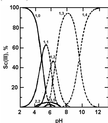
Рис. 3. Діаграма розподілу різних форм \text{Sc}(\text{III}) залежно від \text{pH} розчину: 1,0\text{-Sc}^{3+} ; 1,1\text{-ScOH}^+ ; 1,2\text{-Sc}(\text{OH})_2^+ ; 1,3\text{-Sc}(\text{OH})_3^0 ; 1,4\text{-Sc}(\text{OH})_4^- ; 2,2\text{-Sc}_2(\text{OH})_2^{4+} ; 3,5\text{-Sc}_3(\text{OH})_5^{4+} (C_{\text{Sc}(\text{III})} = 10^{-5} \text{ M})
