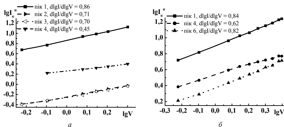
Рис. 4. Залежності критерію Семерано для катодних піків нітрованого Тр О (а) та нітрованого дисазобарвника (б). C_{HCl} = 0,5 М, C_{NaNO_2} = 1,25 \cdot 10^{-2} М, C_{СДМ} = 3,9 \cdot 10^{-5} М, C_{TrO} = 6,0 \cdot 10^{-5} М, C_{Na_2B_4O_7} = 0,01 М, рН = 10,5, V = 1,0 В/с.
