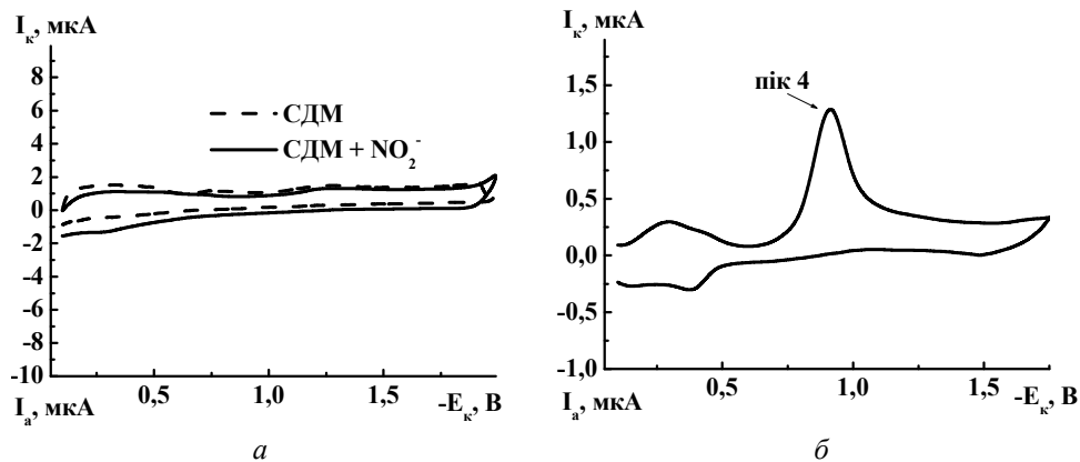
Рис. 2. Циклічні вольтамперограми розчинів СДМ за наявності та без натрій нітриту (а) та Tr O (б). C_{\text{HCl}} = 0,5 \text{ M} , C_{\text{СДМ}} = 1,3 \cdot 10^{-5} \text{ M} , C_{\text{NaNO}_2} = 1,25 \cdot 10^{-2} \text{ M} , C_{\text{TrO}} = 2,5 \cdot 10^{-5} \text{ M} , C_{\text{Na}_2\text{B}_4\text{O}_7} = 0,01 \text{ M} , \text{pH} = 10,5 , V = 1,0 \text{ V/c} .
