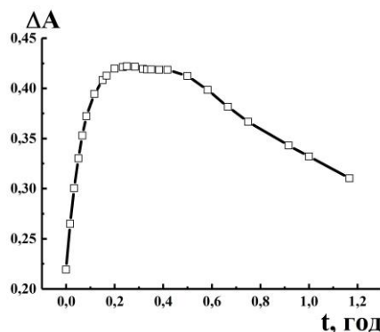
Рис. 7. Стабільність у часі світлопоглинання продукту азосполучення ДНСК з ОТЦ. C_{\text{ДНСК}} = 3,75 \times 10^{-4} \text{ M} ; C_{\text{ОТЦ}} = 1,5 \times 10^{-4} \text{ M} ; C_{\text{NaOH}} = 10,0 \text{ M} ; \lambda_{\text{max}} = 470 \text{ нм} ; l = 1 \text{ см} Fig. 7. Effect of the keeping time on the absorbance of azocoupling products of DNSA with OTC. C_{\text{DNSA}} = 3.75 \times 10^{-4} \text{ M} ; C_{\text{OXT}} = 1.5 \times 10^{-4} \text{ M} ; C_{\text{NaOH}} = 10.0 \text{ M} ; \lambda = 470 \text{ nm} ; l = 1 \text{ cm}
