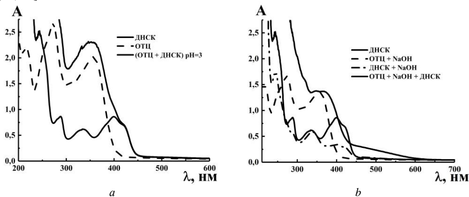
Рис. 2. Електронні спектри поглинання розчинів ДНСК, ОТЦ та продуктів їхньої взаємодії: C_{\text{ДНСК}} = 2,625 \times 10^{-4} М; C_{\text{ОТЦ}} = 1,5 \times 10^{-4} М; C_{\text{NaOH}} = 10,0 М Fig. 2. Absorption spectra of DNSA, OXT solutions and products of their interaction. C_{\text{DNSA}} = 2.625 \times 10^{-4} М; C_{\text{OXT}} = 1.5 \times 10^{-4} М; C_{\text{NaOH}} = 10.0 М
