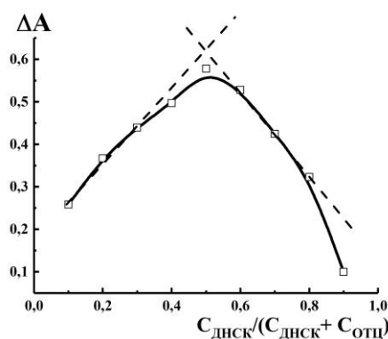
Рис. 6. Визначення співвідношення компонентів у системі ДНСК–ОТЦ методом ізомолярних серій. C_{\text{ДНСК}} + C_{\text{ОТЦ}} = 5,0 \times 10^{-4} \text{ M} ; C_{\text{NaOH}} = 10,0 \text{ M} ; l = 1 \text{ cm} ; \lambda_{\text{max}} = 470 \text{ nm}
