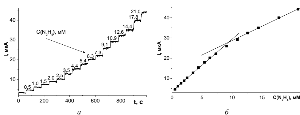
Рис. 4. Амперометричні відклики (за E=+0,6 В та pH 8,2) макета гідразинного сенсора на ПАН/Pd-платформі на додавання розчинів визначуваного субстрату (а) та градувальний графік (б) досліджуваного сенсора для мілімолярного концентраційного діапазону Fig. 4. Amperometric responses (under the E = +0.6 V and pH 8.2) of the model of hydrazine sensor on the PAN/Pd platform to the introduction of the solutions of determined substrate (a) and the calibration graph (b) of studied sensor for the millimolar concentration range
