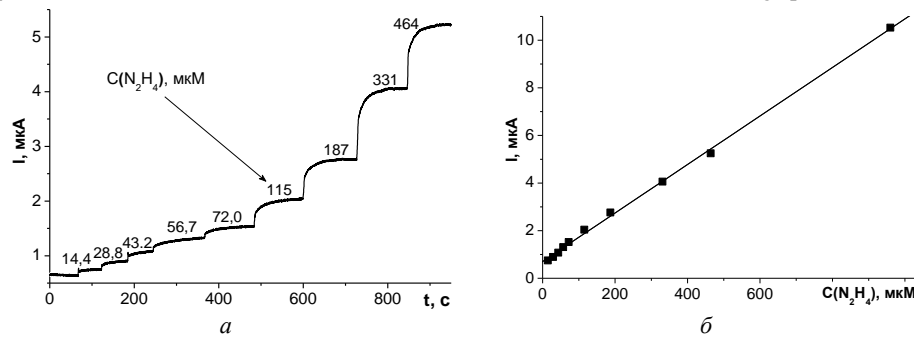
Рис. 7. Амперометричні відклики (за E=+0,6 В та \text{pH } 8,2 ) макета гідразинного сенсора на ПАН/Pd-платформі на додавання розчинів визначуваного субстрату (а) та градувальний графік (б) досліджуваного сенсора для мікромолярного концентраційного діапазону
