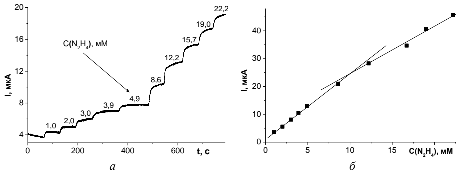
Рис. 6. Амперометричні відклики (за E=+0,55 В та \text{pH } 9,3 ) макета гідразинного сенсора на ПАН/Pd-платформі на додавання розчинів визначуваного субстрату (а) та градувальний графік (б) досліджуваного сенсора
