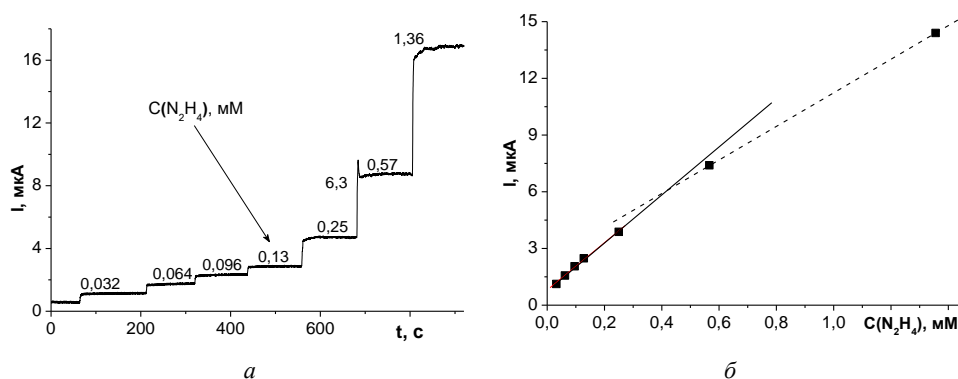
Рис. 5. Амперометричні відклики (за E=+0,55 В та pH 8,8) макета гідразинного сенсора на ПАН/Pd-платформі на додавання розчинів визначуваного субстрату (а) та градувальний графік (б) досліджуваного сенсора Fig. 5. Amperometric responses (under the E = +0.55 V and pH 8.8) of the model of hydrazine sensor on the PAN/Pd platform to the introduction of the solutions of determined substrate (a) and the calibration graph (b) of studied sensor
