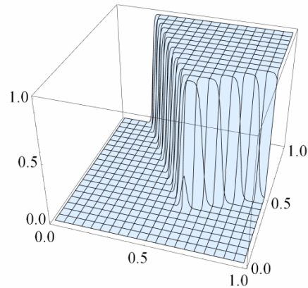
Рис. 2. Точний розв'язок задачі (25)
