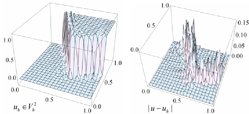
Рис. 3. Ілюстрація результатів розв'язування задачі (25) МСЕ для 20 \times 20 чотирикутних скінченних елементів з квадратичними серендиповими апроксимаціями
